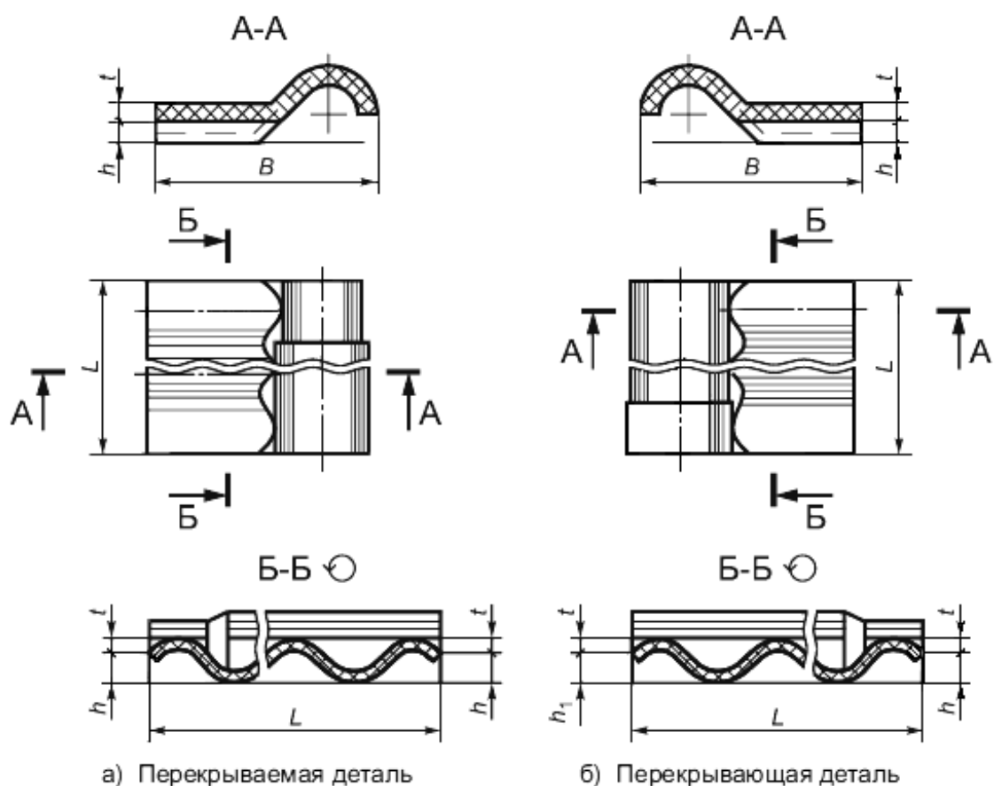
Рисунок 6 - Коньковые детали
