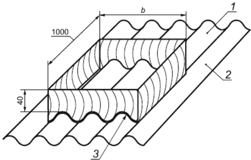
1 - рама; 2 - лист; 3 - герметизирующий материал
