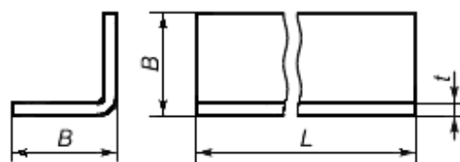
Рисунок 8 - Упрощенные коньковые детали
