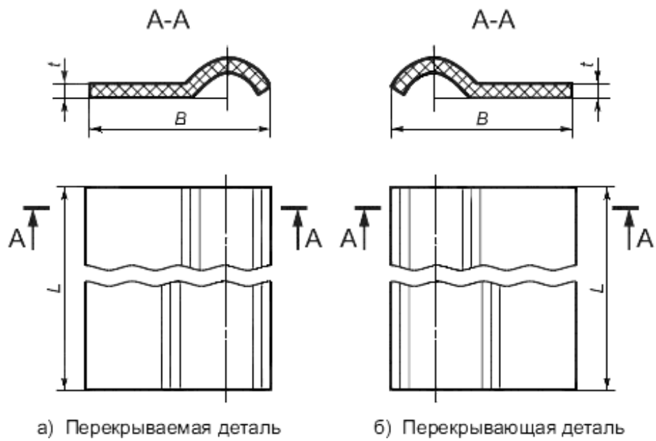
Рисунок 7 - Арочные коньковые детали
